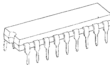
DIP18-P-300-2.54D
