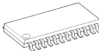
SSOP24-P-300-1.00
