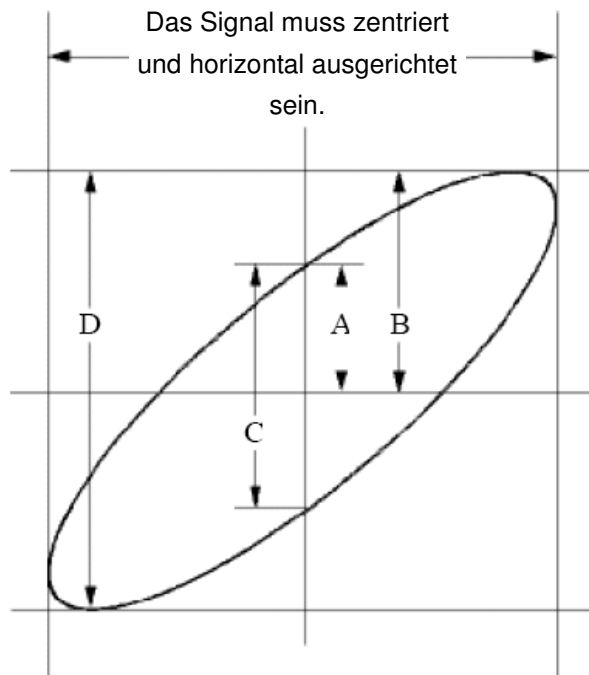
Abb. 84 Lissajous-Figur
