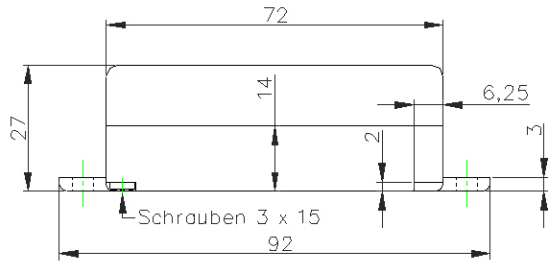
Gehäuseoberteil mit Unterteil verschraubt
