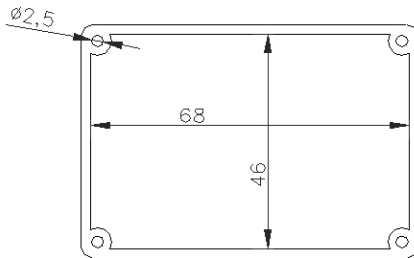
Klarsicht – Gehäuseoberteil
