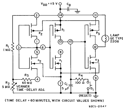
Fig. 26—Analog timer using CA3600E.
