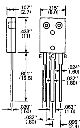
Fig. T67 TO-126M ECG 2504
